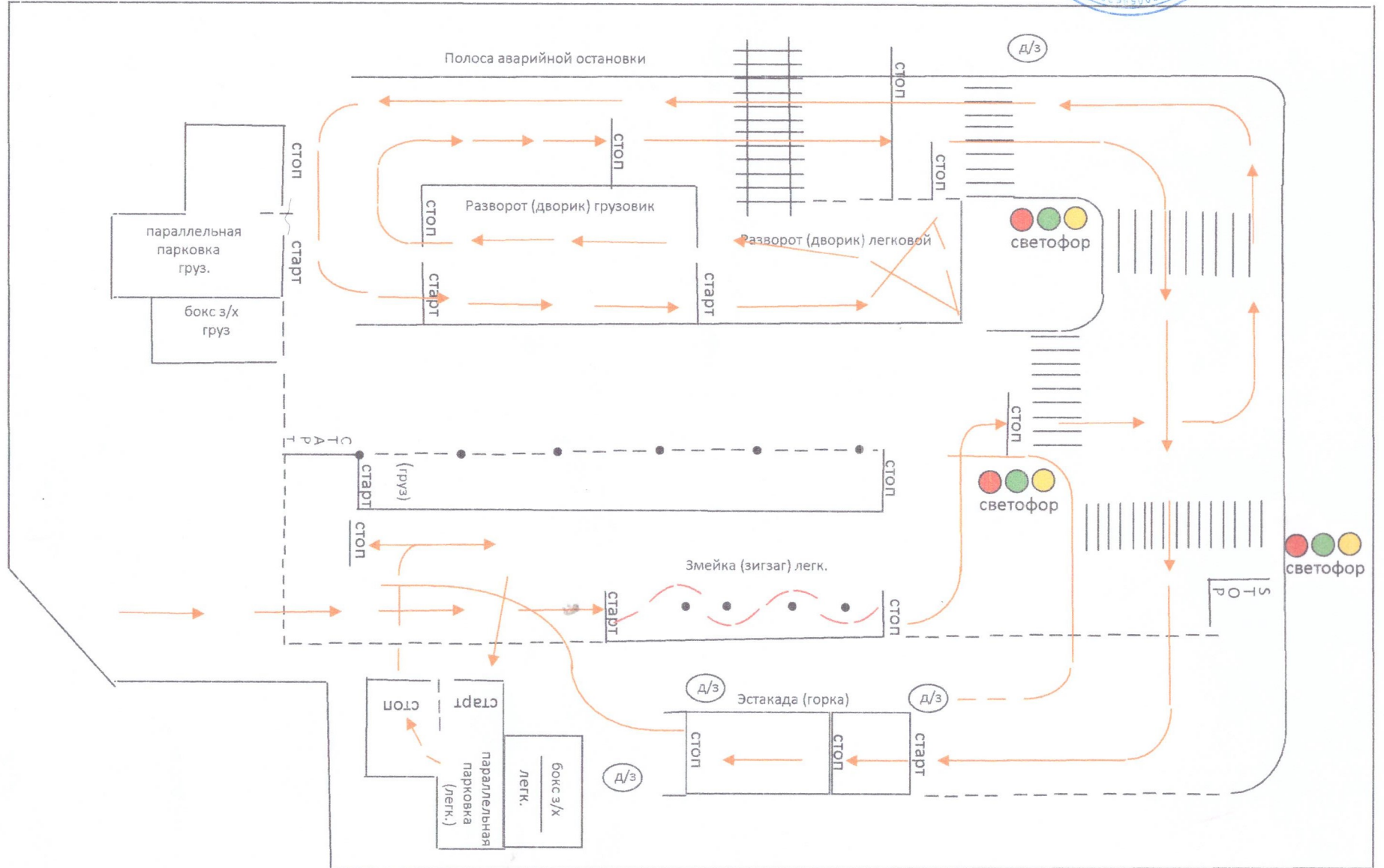
Схема маршрута движения легкового автомобиля на полигоне ГБПОУ «ДМТ»
